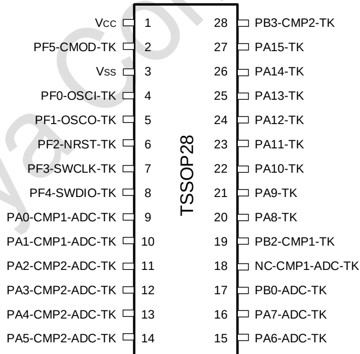
图 3-2 TSSOP28 Pinout4 PY32T020G4xP7-B (Top view)
