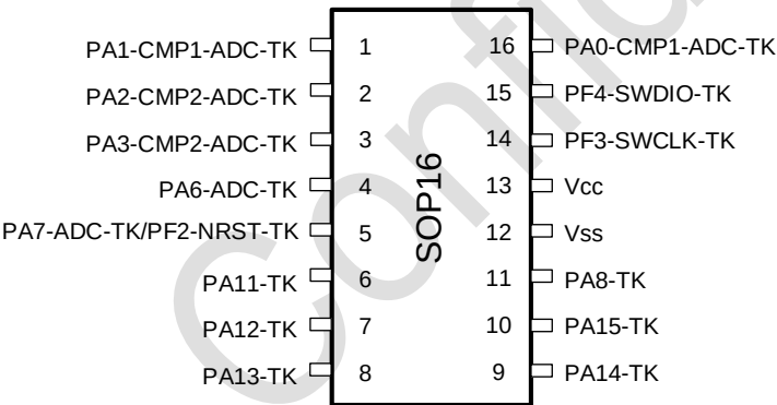
图 3-11 SOP16 Pinout2 PY32T020W2xS7-B (Top view)
